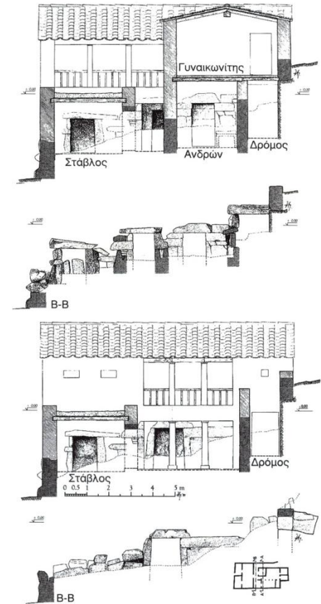
Δόσιος. Απόψεις και τομές των τοίχων (με κατεύθυνση από τα ανατολικά προς τα δυτικά) του κεντρικού τμήματος της οικίας. Κλίμακα 1:200.
