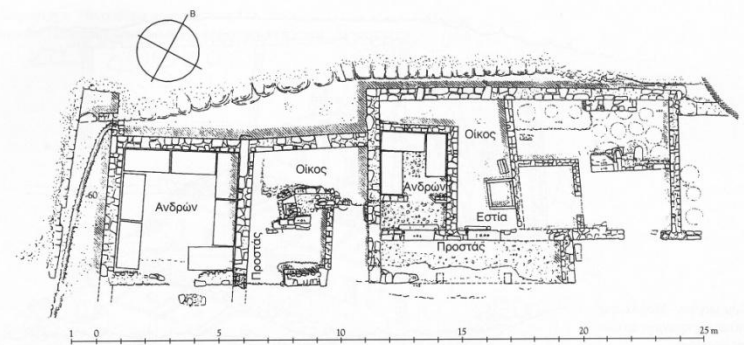
Ξώβουργο. Μονόκωρα οπίτα μετά την ενσωμάτωση των ανδρώνων και με έναν ανδρώννα ο οποίος κατασκευάστηκε μόλις τον 5ο αιώνα.
