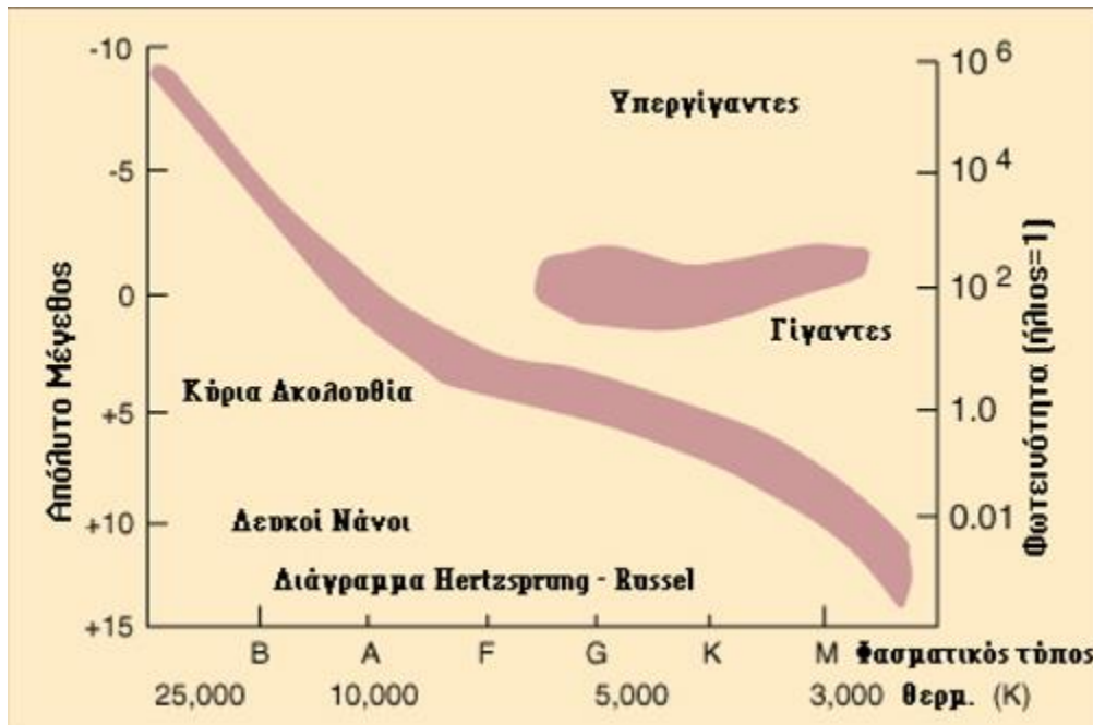
Διάγραμμα H-R
