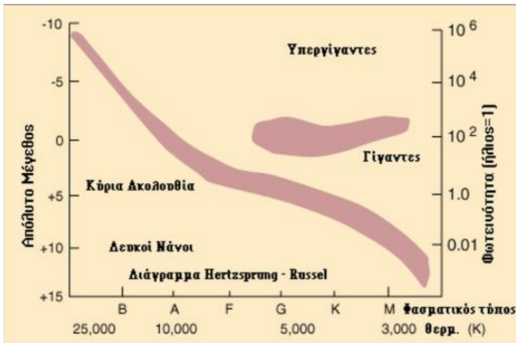
Διάγραμμα H-R
